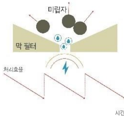
플라즈마필터의 입자처리 개념도
